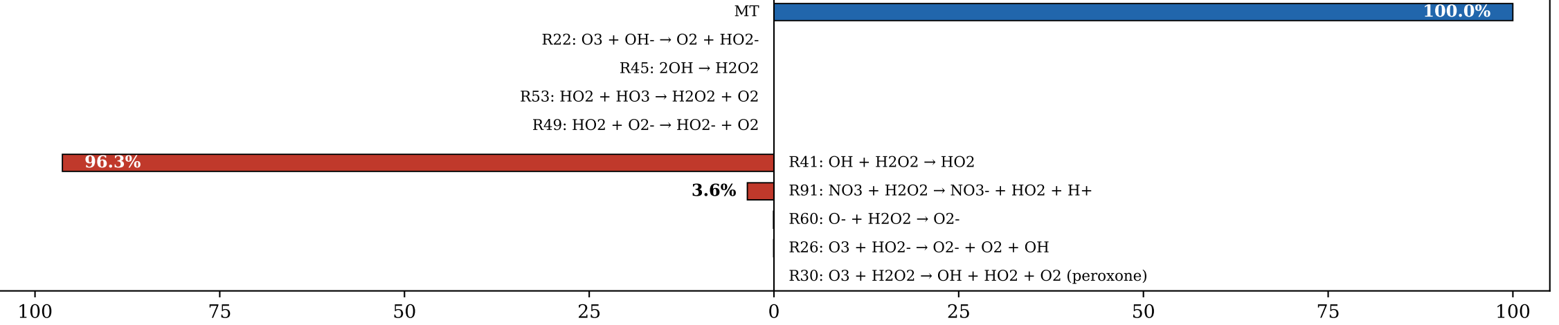
(d) H 2 O 2 (Σsrc = 1.79e-08 M/s)
